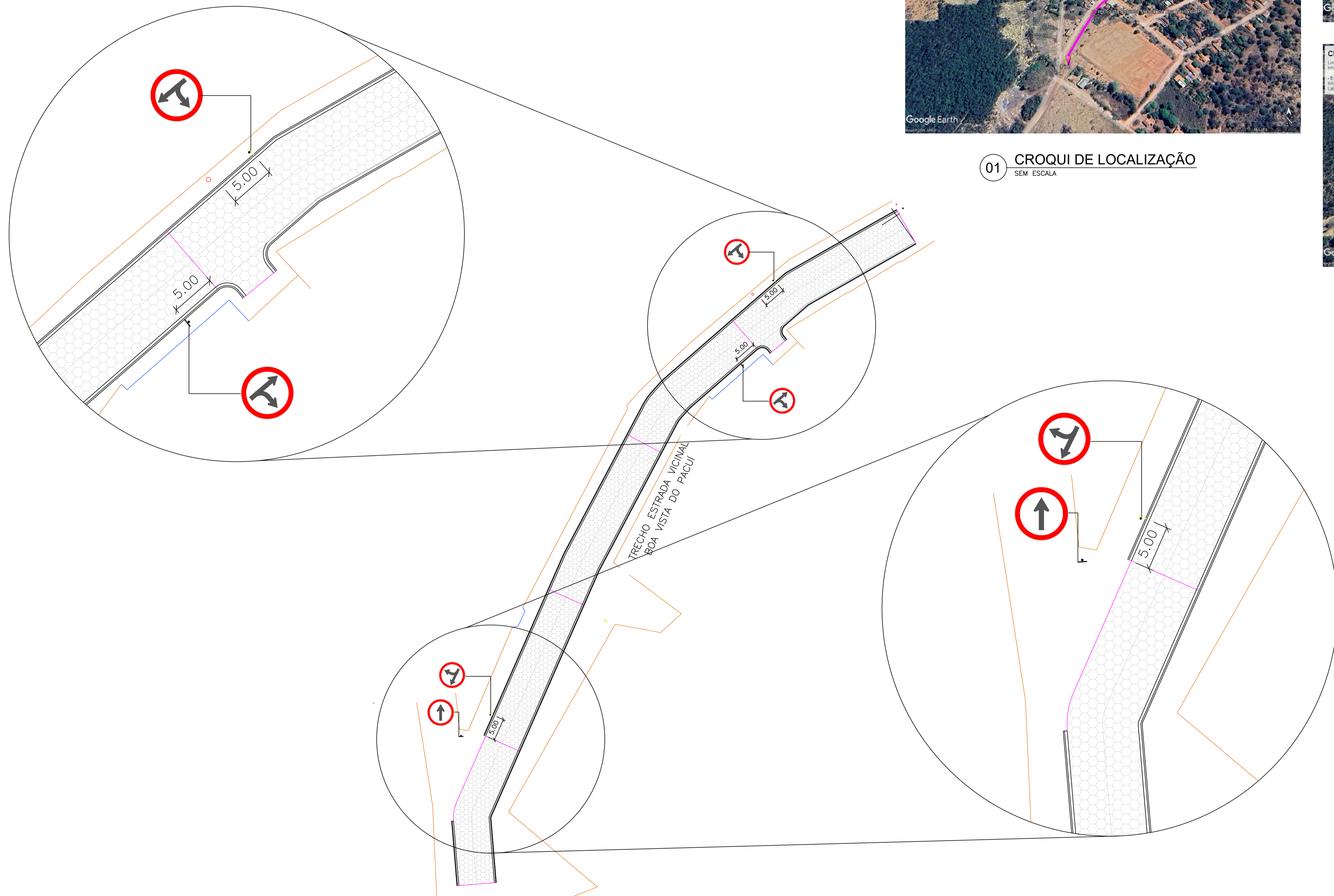
02 PROJETO DE SINALIZAÇÃO DO TRECHO DA ESTRADA VICINAL DE BOA VISTA DO PACUÍ 1:500
