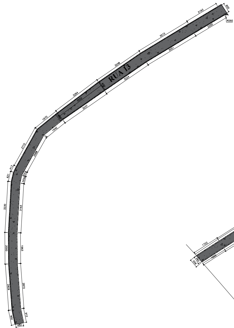
PAVIMENTAÇÃO ESC 1/100
