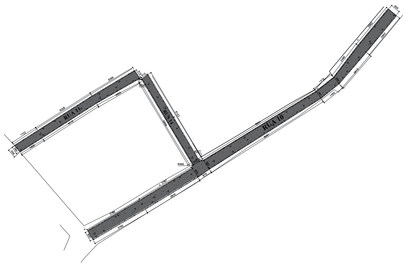
PAVIMENTAÇÃO ESC 1/100
